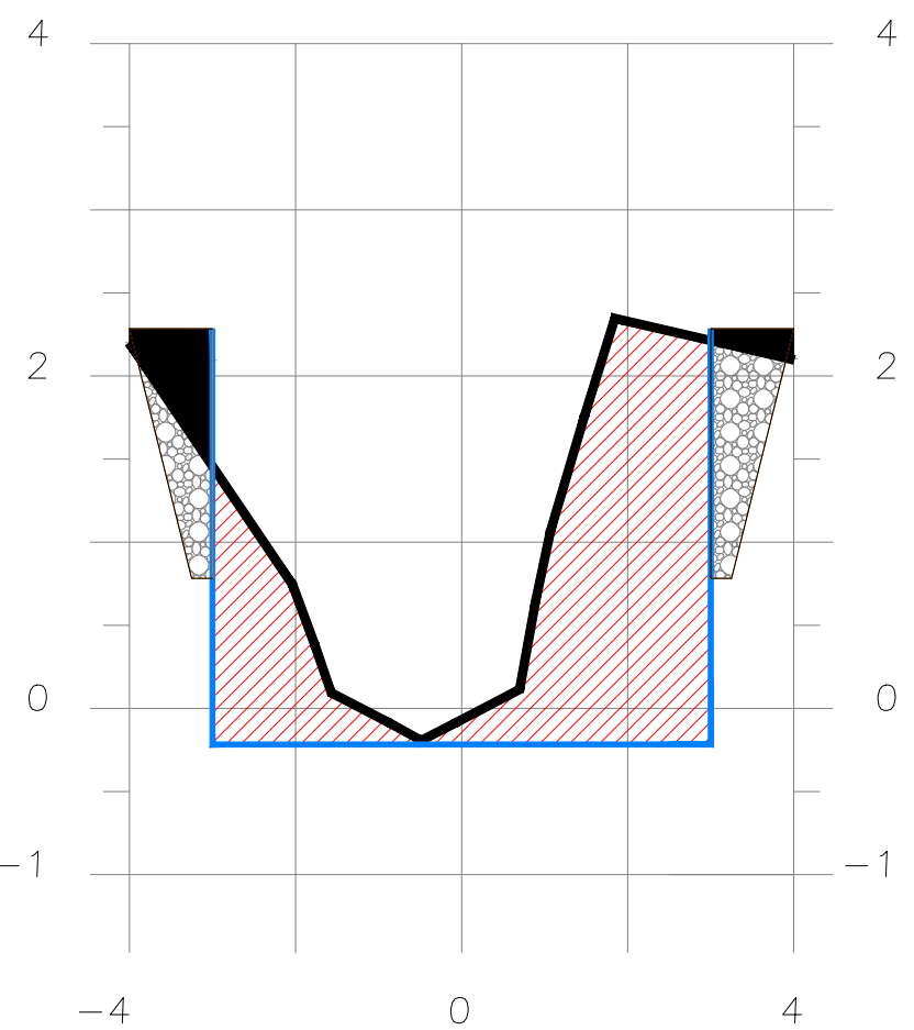
SECCION 2+265
