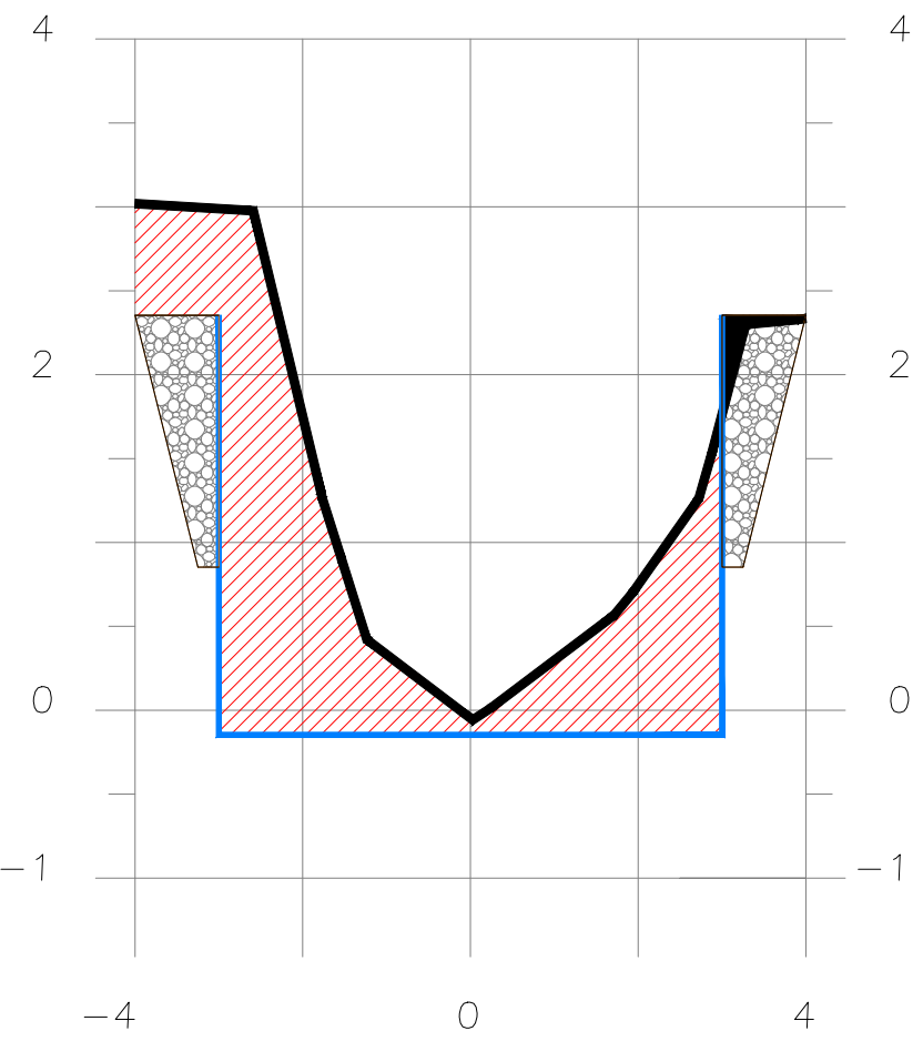
SECCION 2+100
