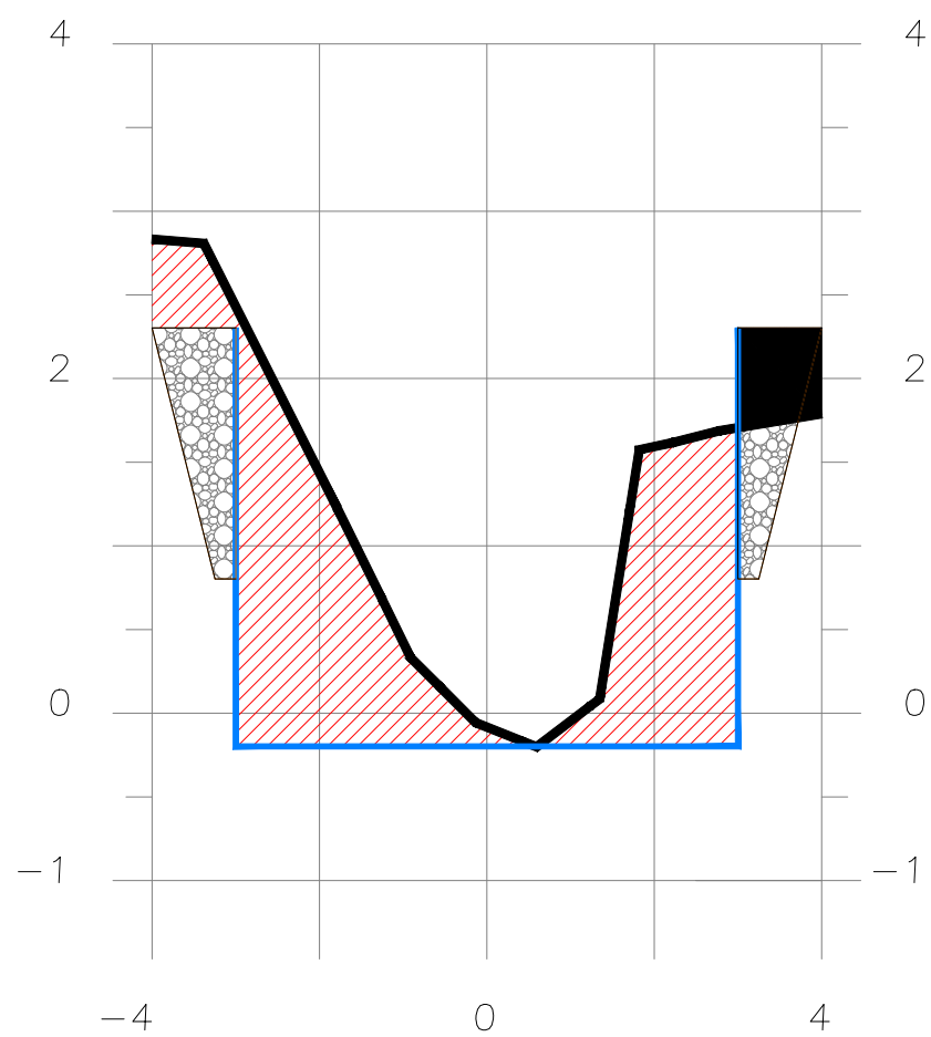
SECCION 2+200
