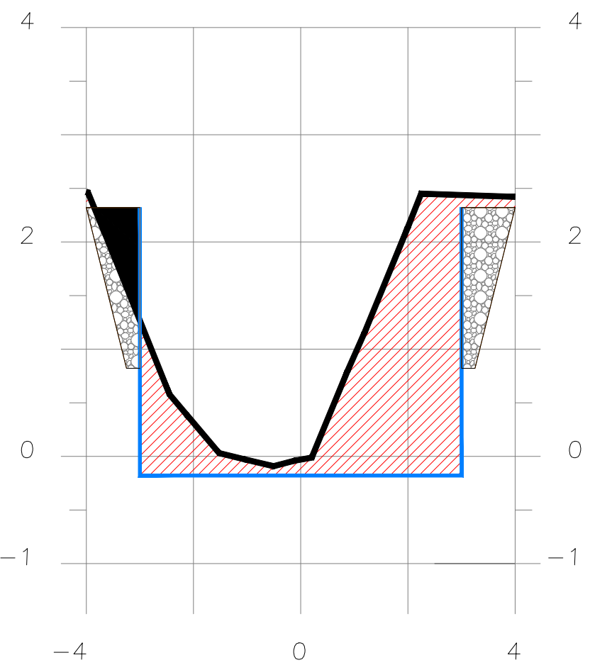
SECCION 2+175
