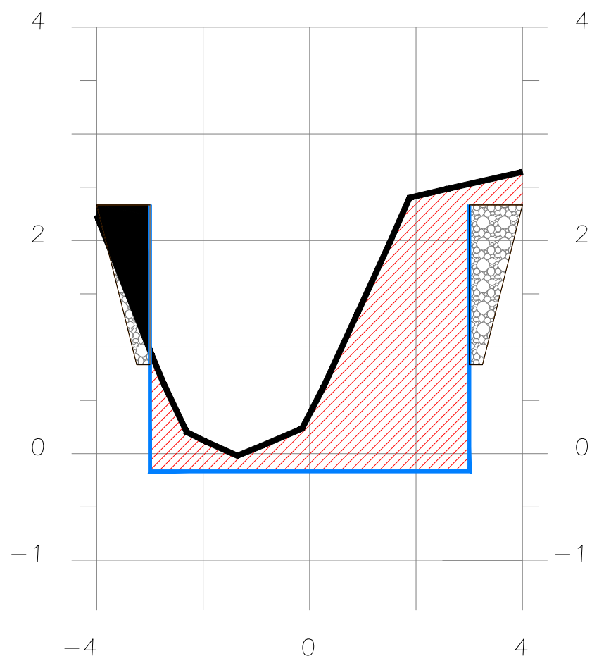
SECCION 2+145
