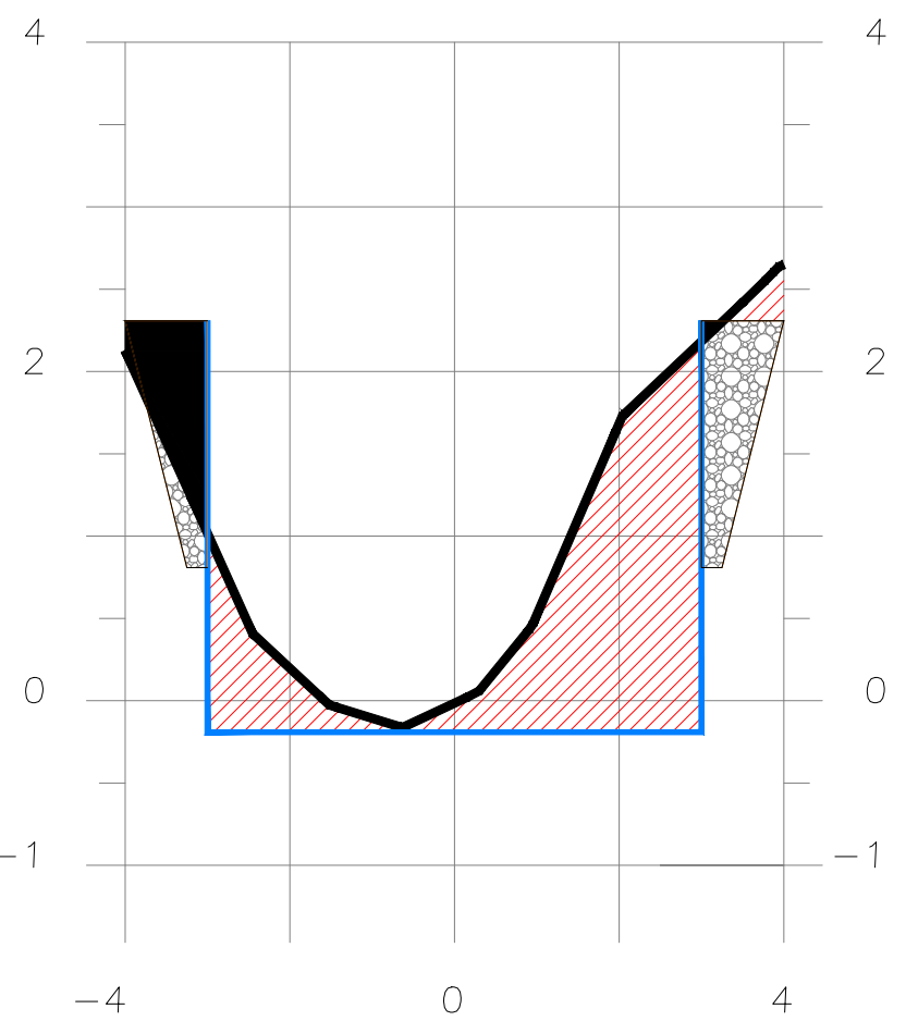
SECCION 2+205
