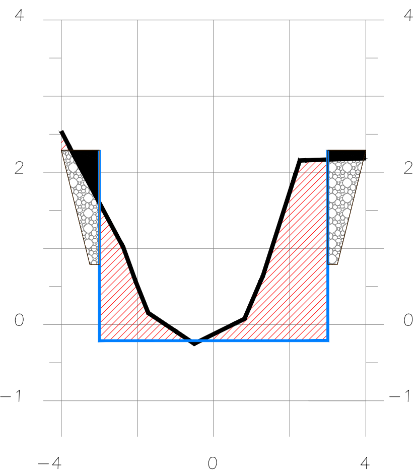
SECCION 2+250
