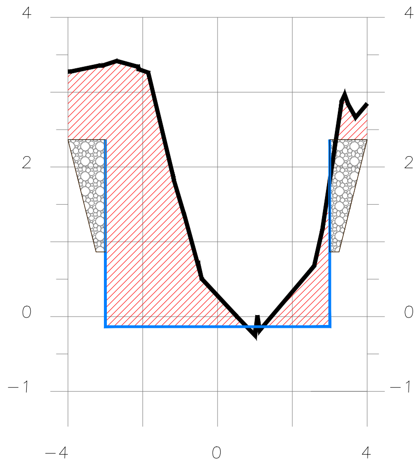
SECCION 2+072.89
