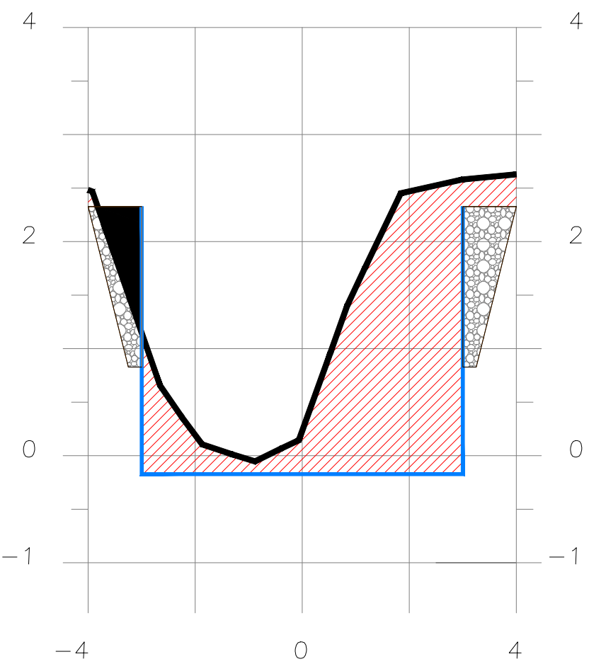
SECCION 2+160
