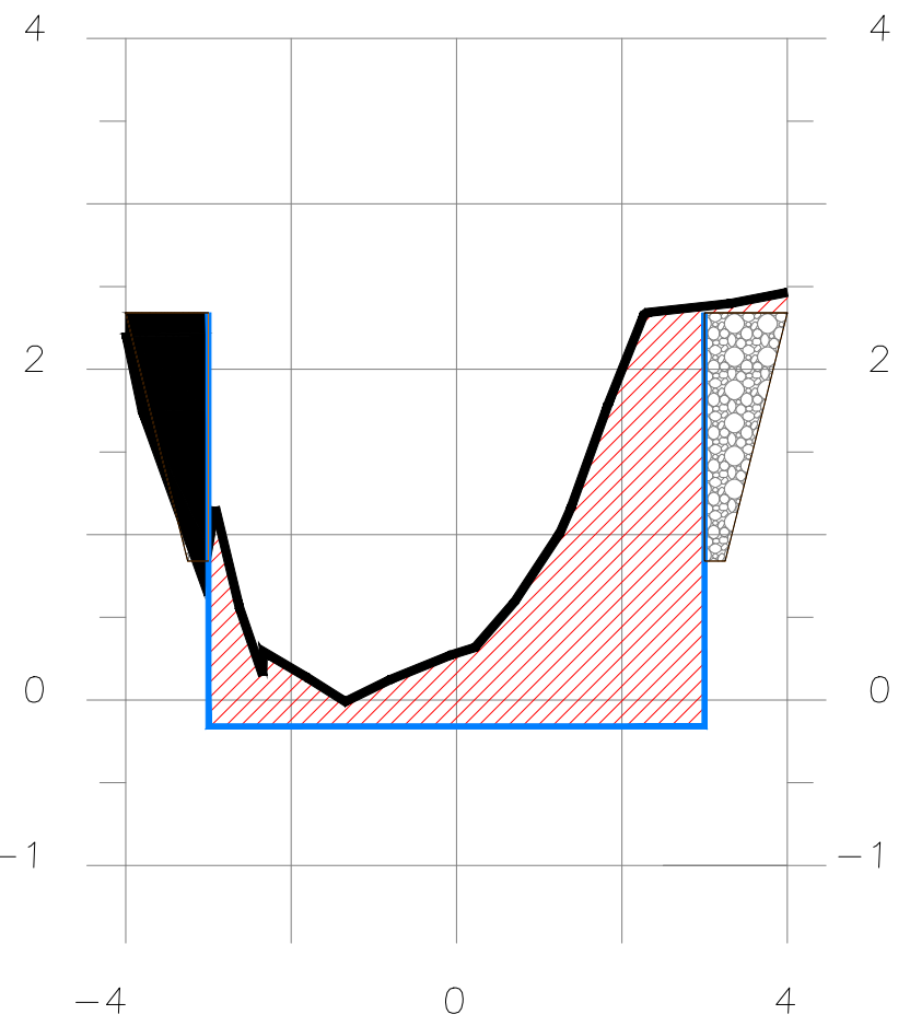
SECCION 2+130
