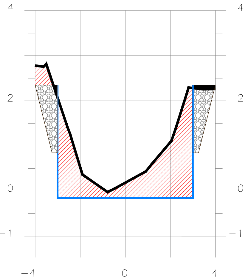
SECCION 2+115
