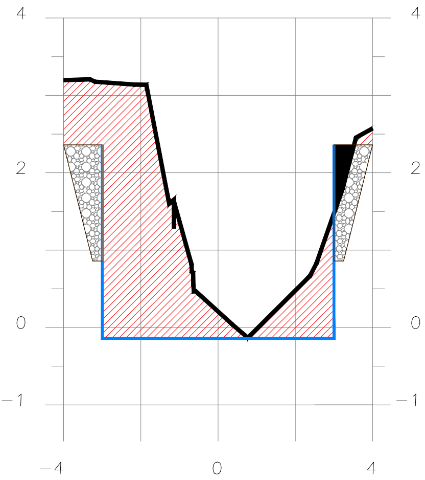
SECCION 2+085
