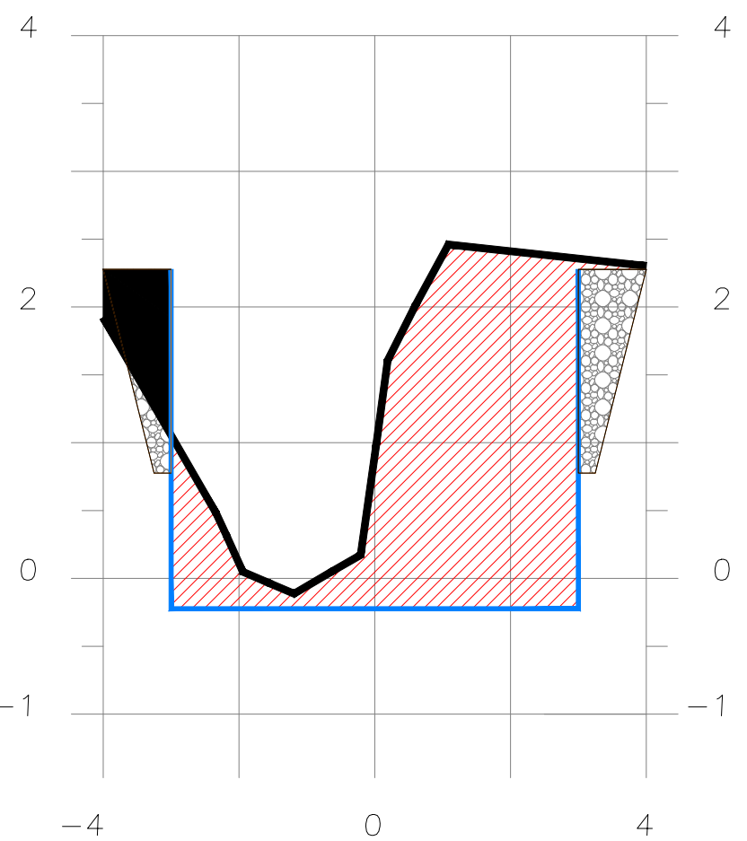
SECCION 2+280
