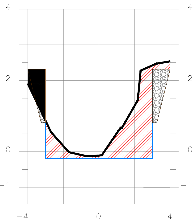
SECCION 2+190
