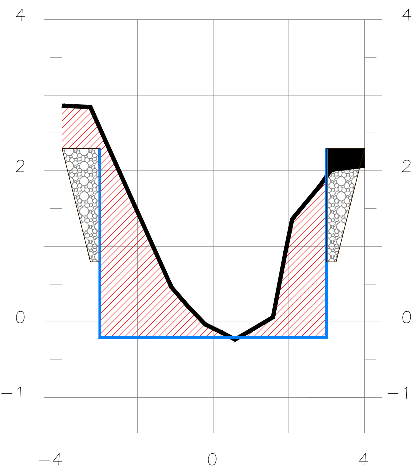
SECCION 2+235
